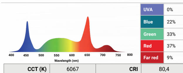
helioSPEC R60F
